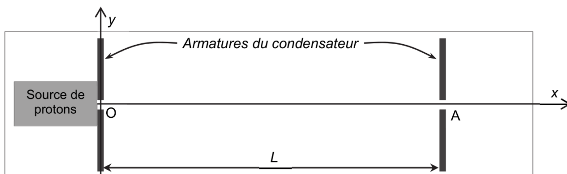
Figure 1. Schéma du dispositif modélisant l'accélérateur linéaire
