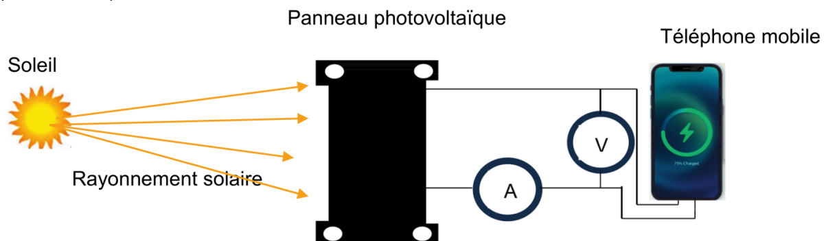
Figure 2. Schéma de l'expérience de charge du téléphone mobile à l'aide du panneau solaire. Un chronomètre permet de suivre l'évolution de la charge de la batterie au cours du temps
